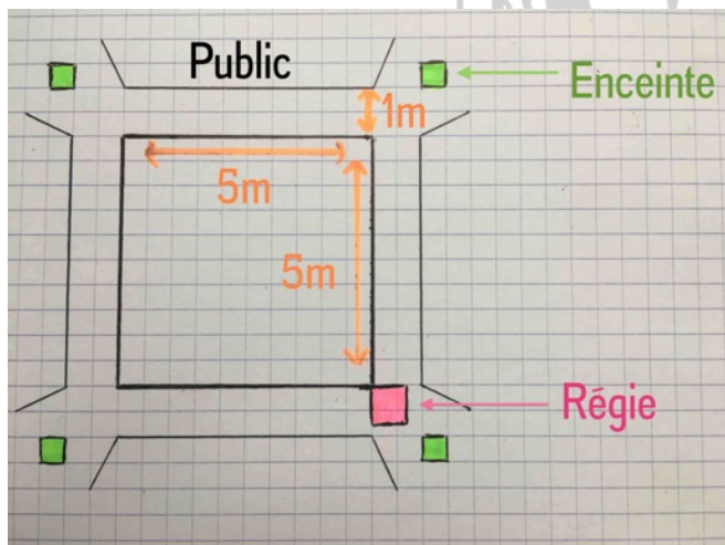
Plan d'implantation
