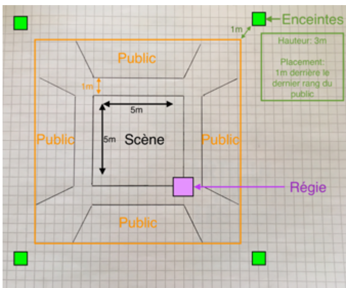
Plan d'implantation
